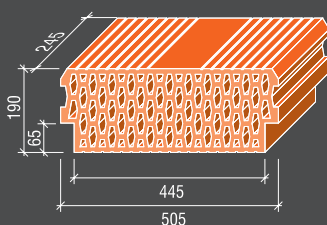
Keramická stropná vložka KSV TermoBRIK - 19/60 počet kusov na palete: 70
